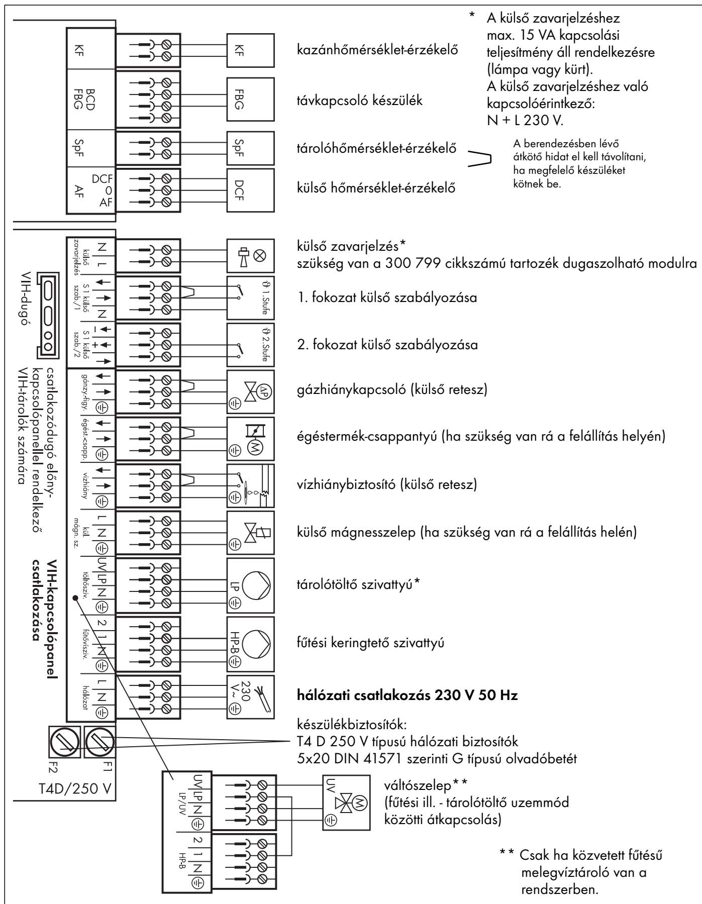
ábra 6.1 Elektromos csatlakozások
