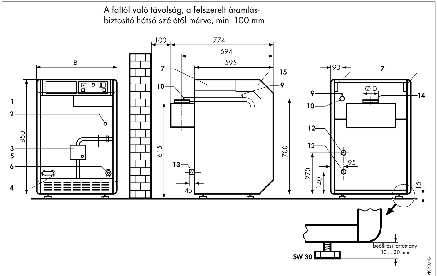
ábra 4.1 Méretek
