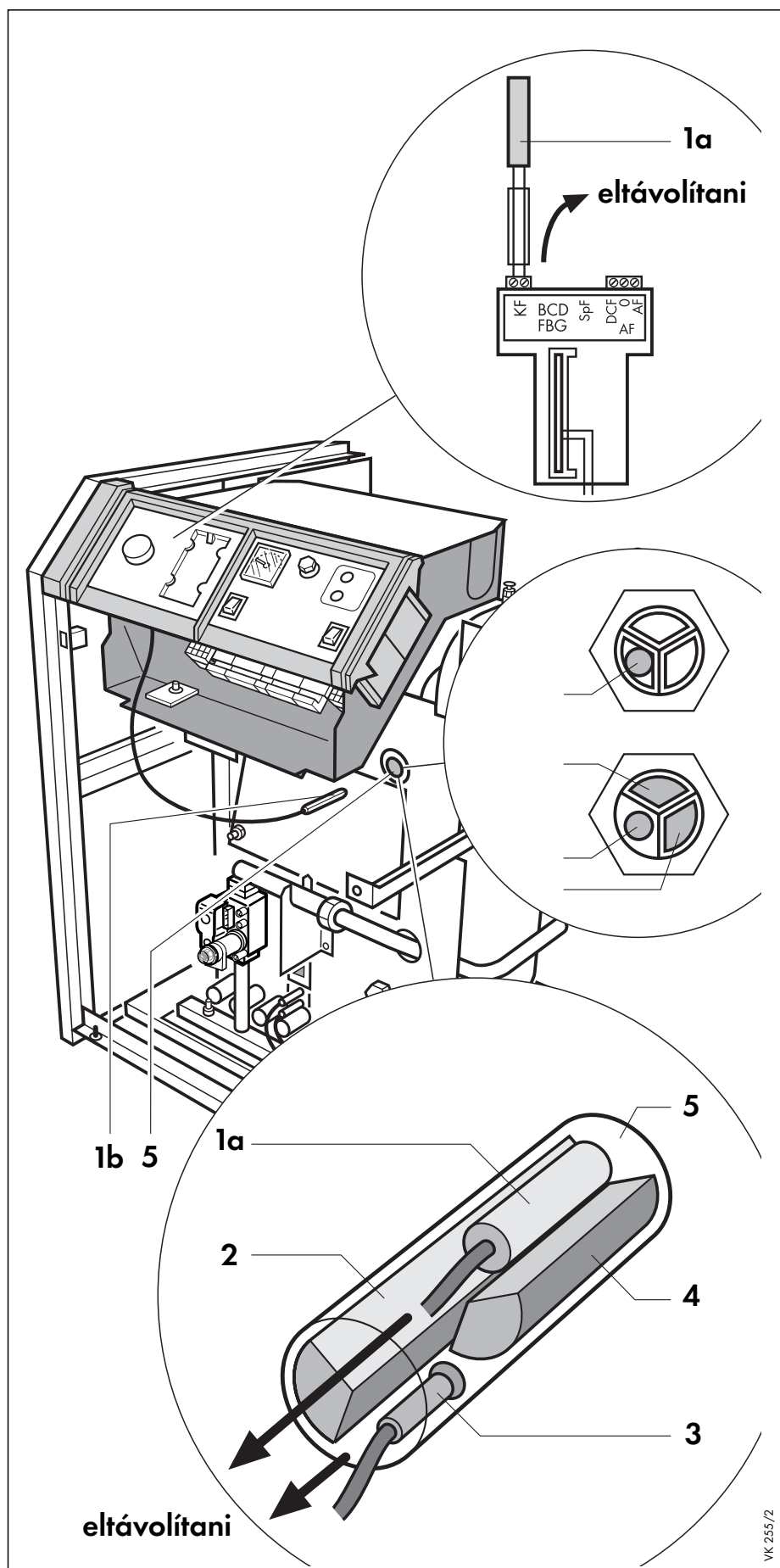
ábra 6.6 Védőhüvely
