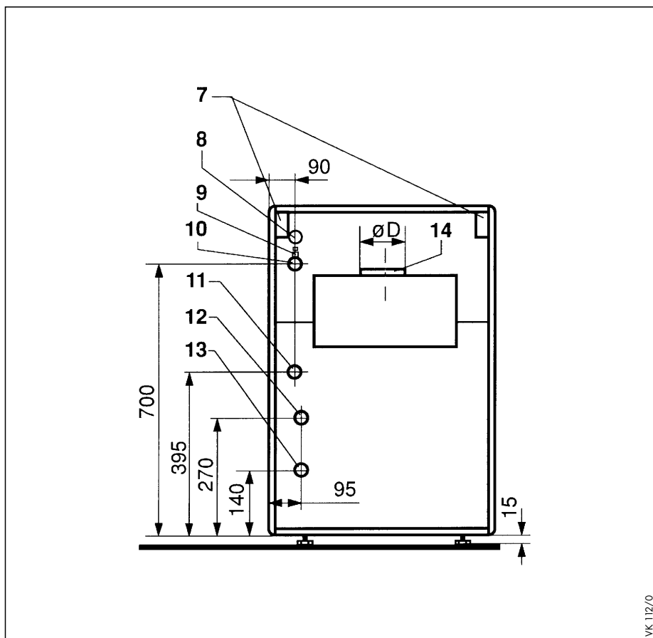
ábra 5.9 Fűtésoldali csatlakozók
