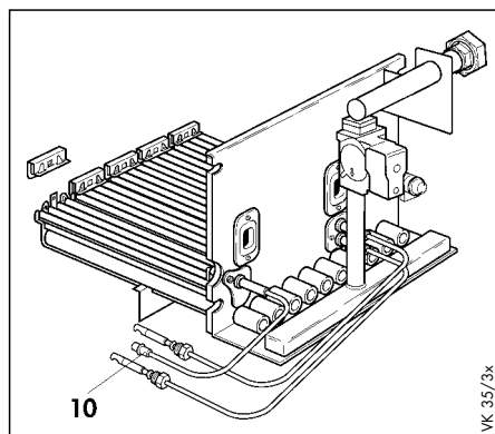
ábra 8.2 A fűvókanyomás mérőcsenkja (VK 32-47)
