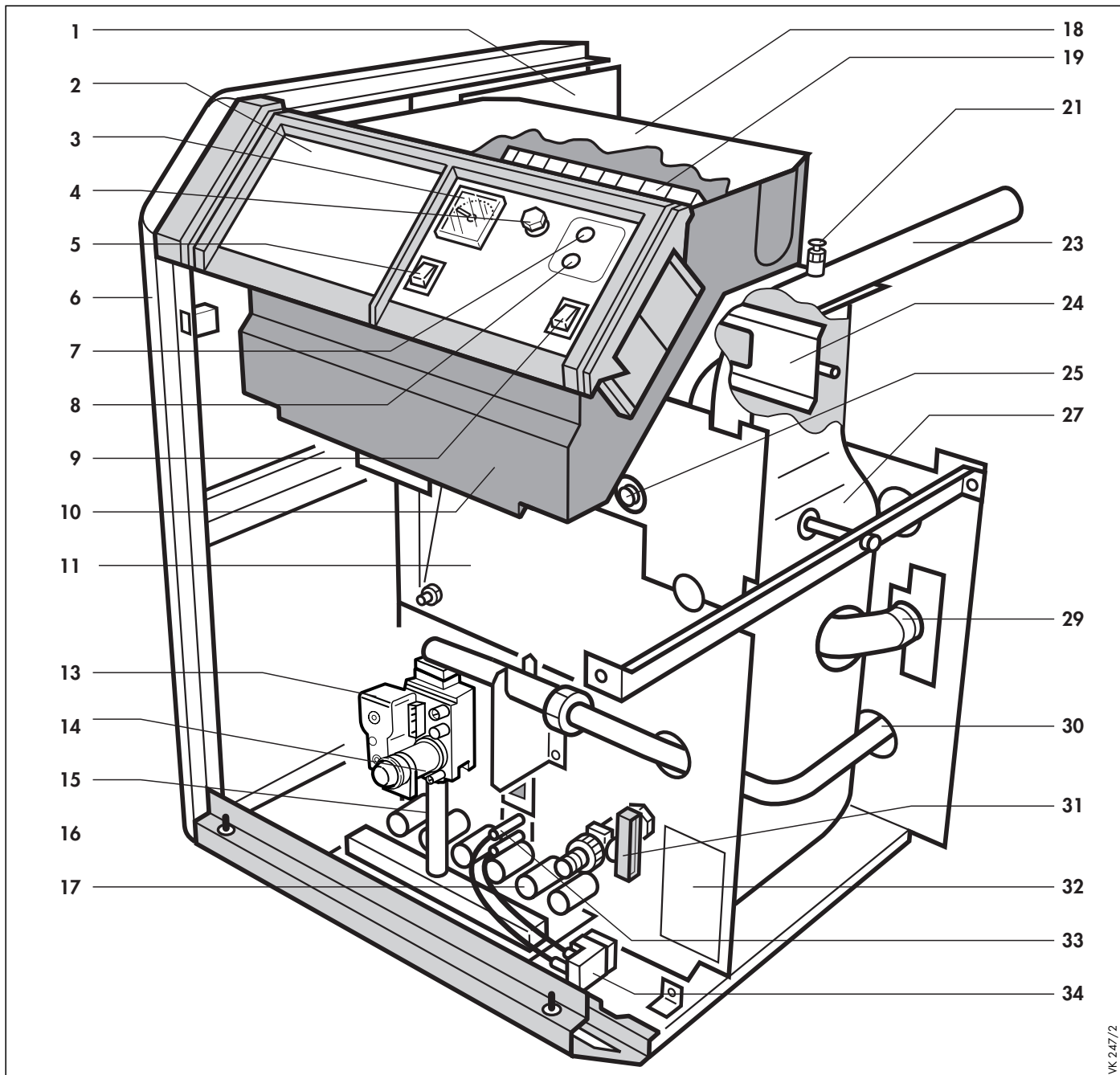
ábra 1.1 A kazán funkcionális részei
