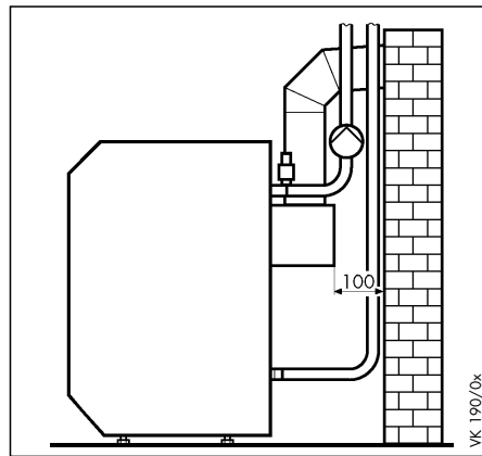
ábra 5.2 Pompcémbem loaoáallított felállítási hely
