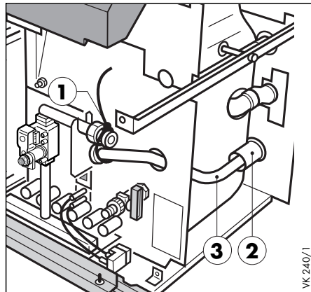
abra 5.6 Gázcsatlakozó cső
